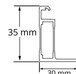
長辺フレーム断面形状
