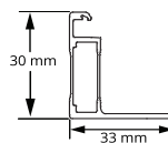
長辺フレーム断面形状
