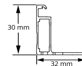
長辺フレーム断面形状
