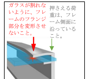
図 1a: クランプで押える荷重の位置
