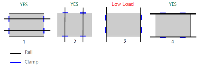
図 3. 架台の構成
