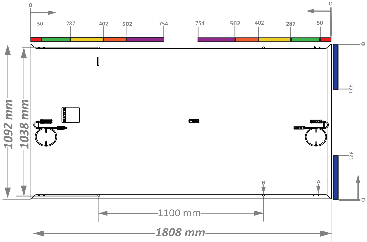
A - 接地穴 (4X Ø 4.2mm) B - フレーム取付穴 (4X 9mm (W) x 14mm (L), R4.5mm)
