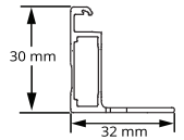
短辺フレーム断面形状
