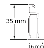
短辺フレーム断面形状
