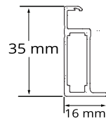
短辺フレーム断面形状
