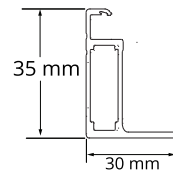
長辺フレーム断面形状
