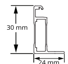
短辺フレーム断面形状
